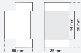
Hutschiene montage 2 TE
